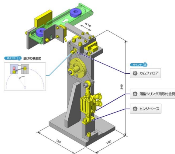
リンクを利用したストップ機構のユニット事例
