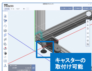
複数溝のアルミフレームにキャスターが取付け可能
