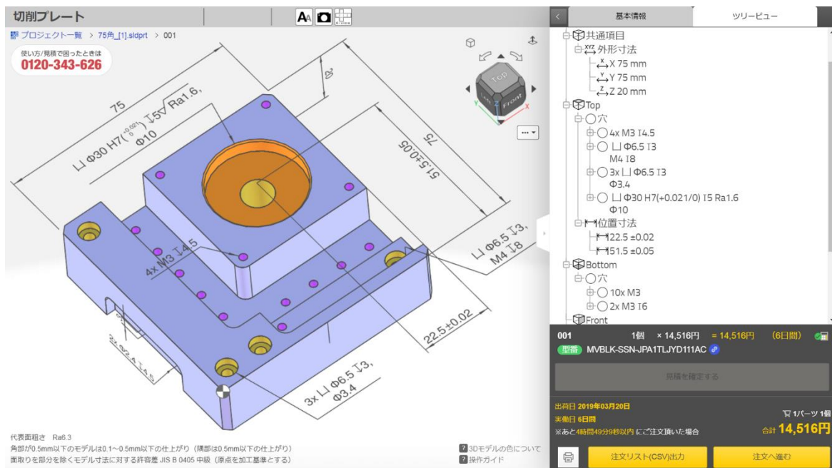
meviy 切削プレートサービスの画面イメージ
